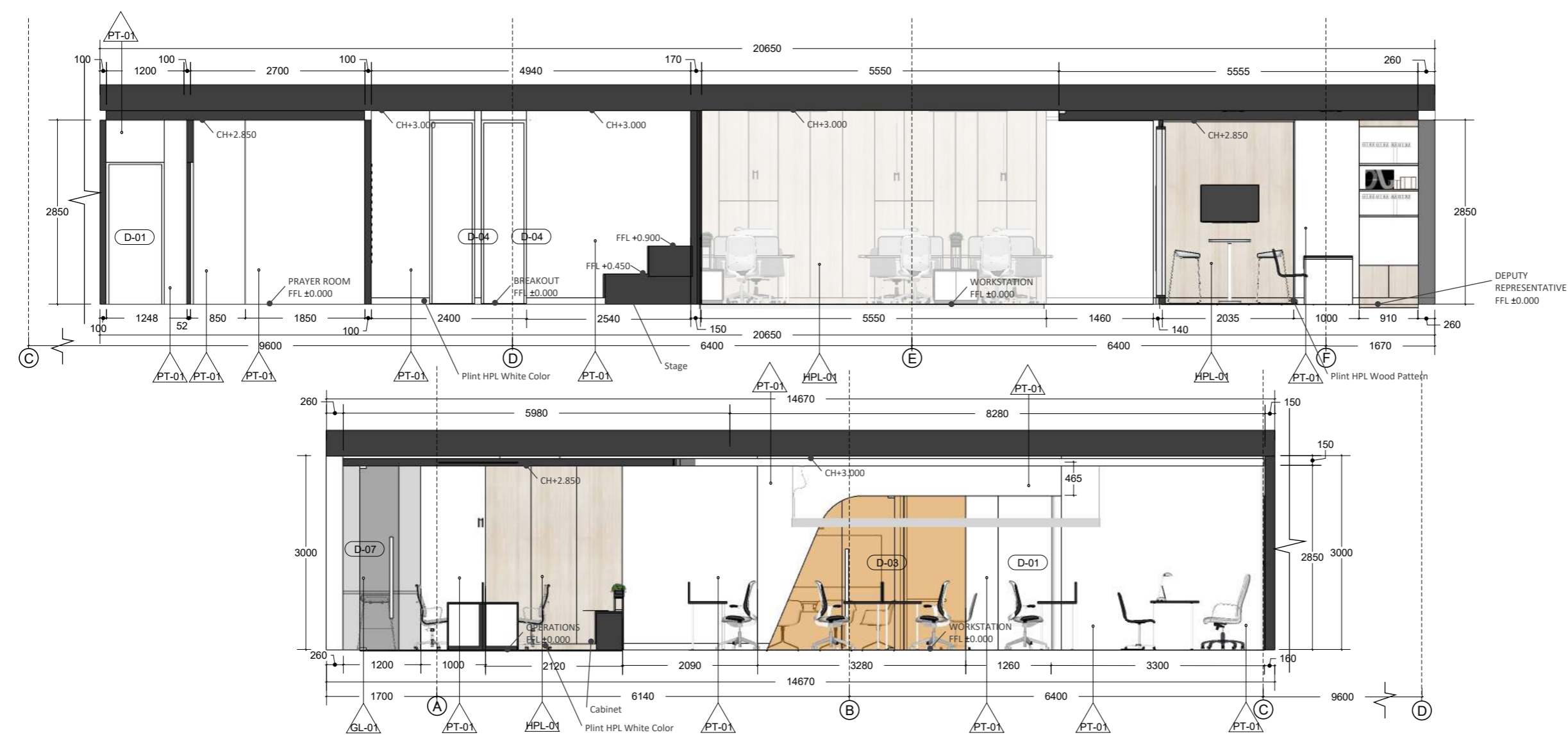
02 Section E INT-202 Scale: 1:75
