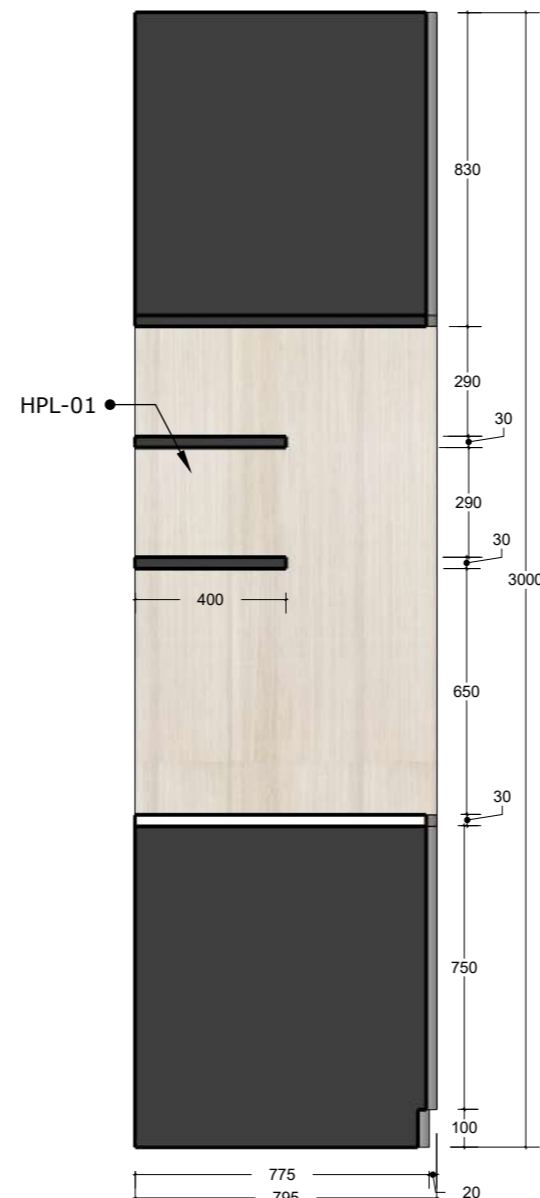
04 SECTION A INT-509 Scale: 1:20
