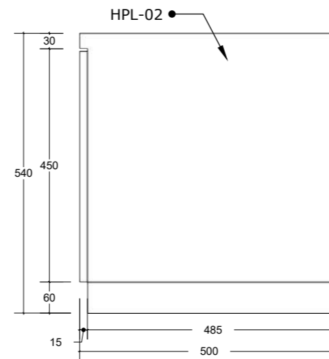
05 RIGHT VIEW INT-512 Scale: 1:10
