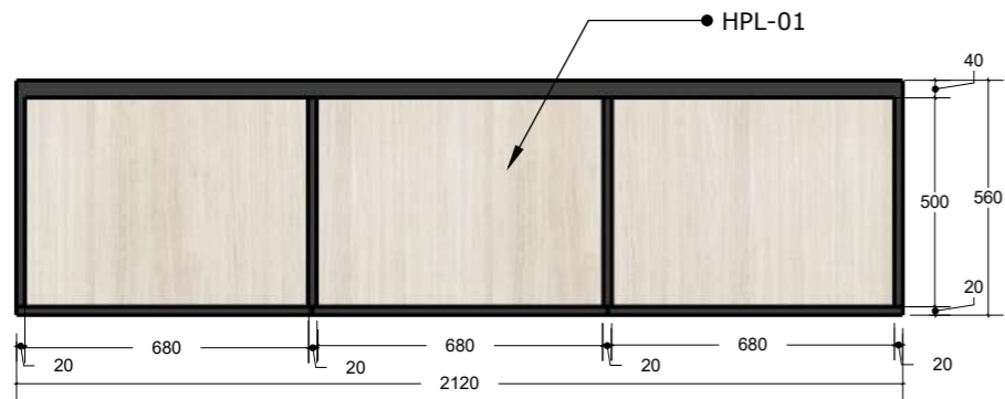
01 SECTION X INT-513 Scale: 1:20
