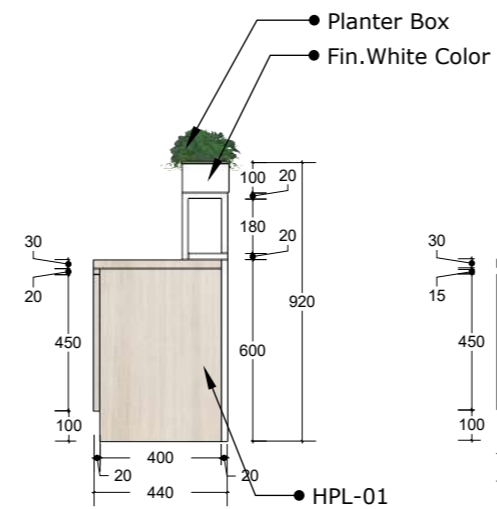
04 RIGHT VIEW INT-514 Scale: 1:25
