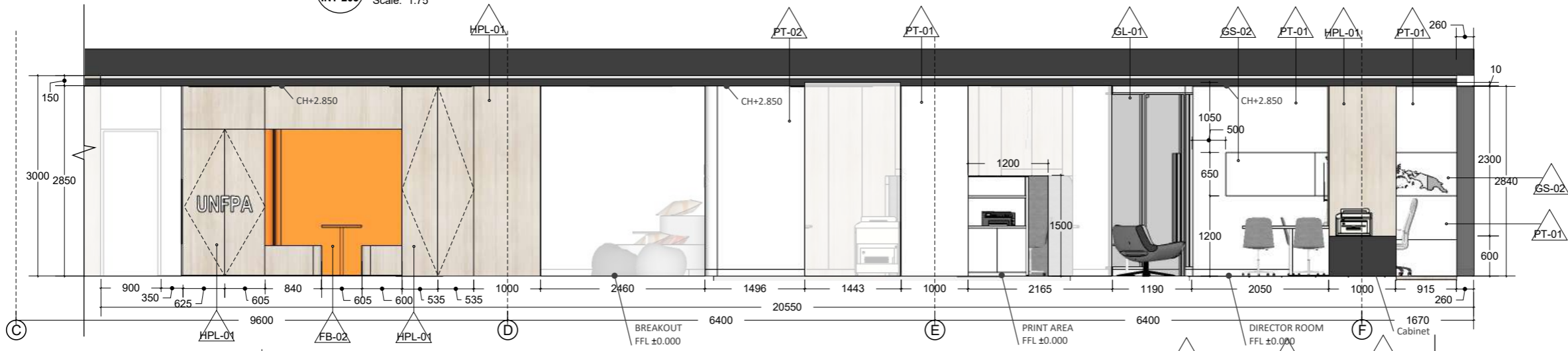
01 Section F INT-203 Scale: 1:75
