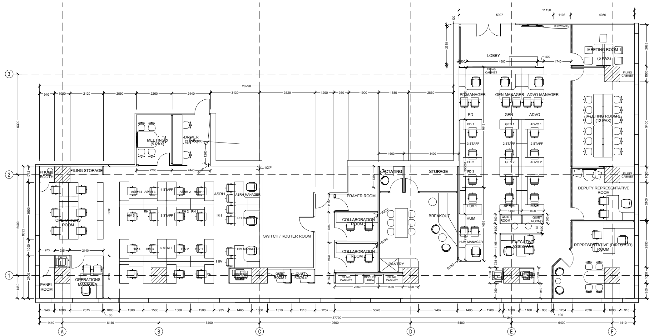
— LAYOUT PLAN INT-101 SCALE 1 : 150
