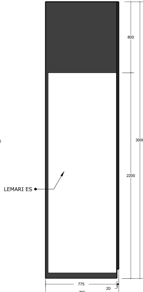
05 SECTION B INT-509 Scale: 1:20
