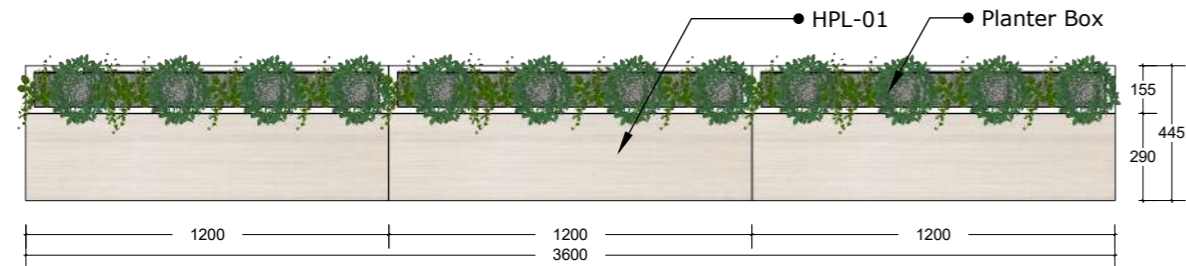
01 TOP VIEW INT-514 Scale: 1:25
