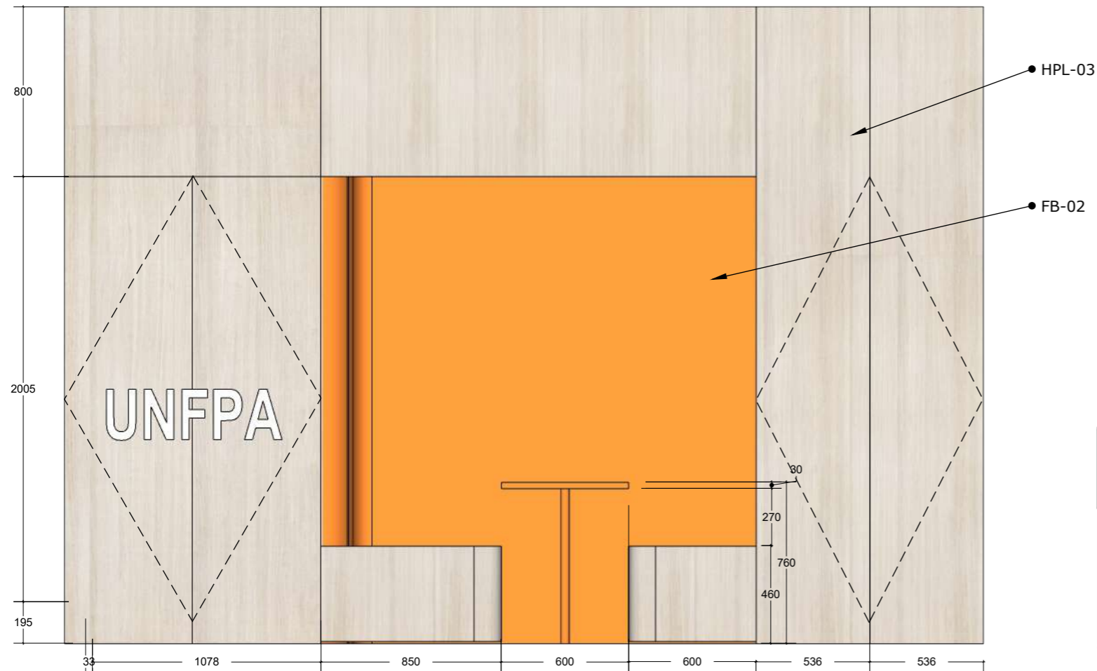
01 FRONT VIEW INT-510 Scale: 1:50
