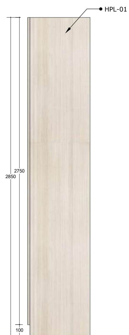
05 RIGHT VIEW INT-513 Scale: 1:20
