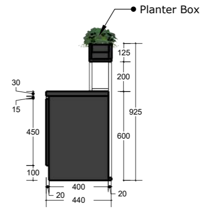
05 SECTION A INT-514 Scale: 1:25
